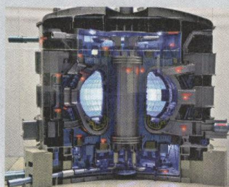
O ITER mostrou, em 2013, uma pequena réplica do reator que está a ser construído no sul de França. O projeto contempla 'portas' para a câmara de confinamento, a pensar também na manutenção
